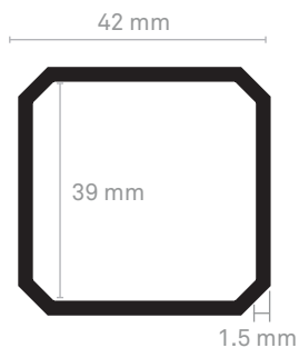
Poste esquinero
